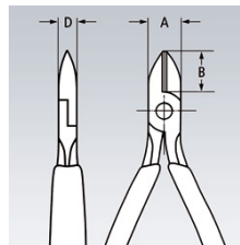
Geschraubtes Gelenk
