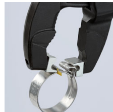
Schließen einer Schlauchselle ohne Anschlag
