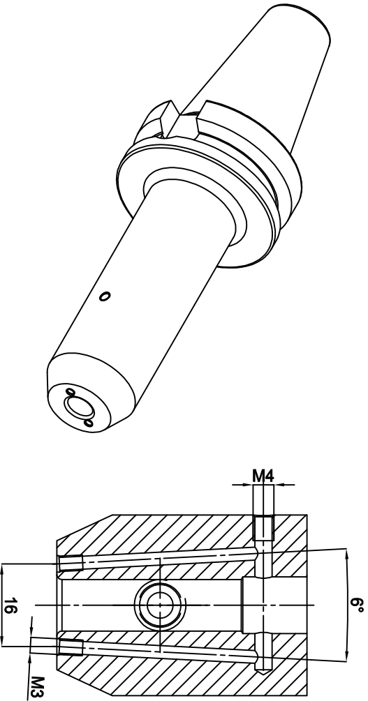
A-A (2:1)
