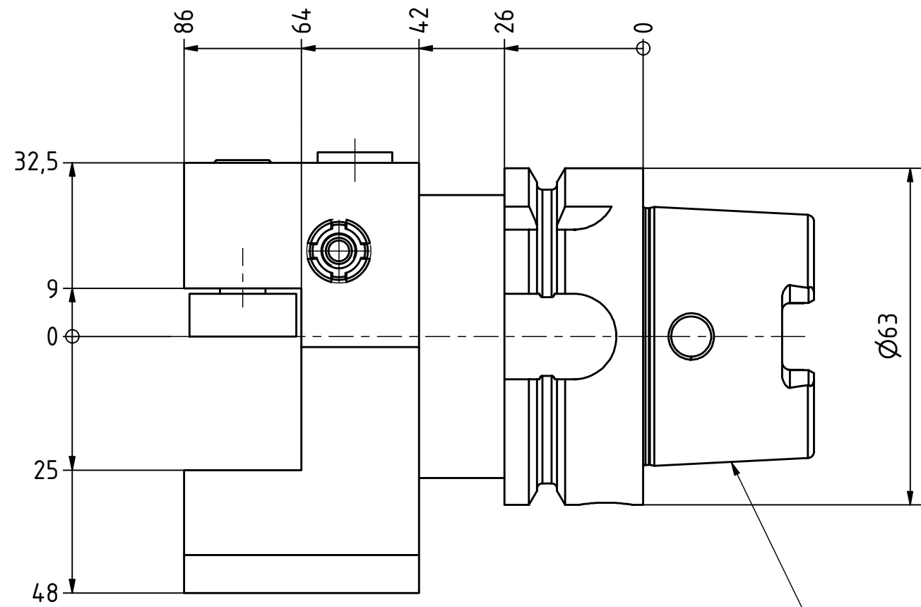
HSK A63 DIN69893 Ausführung T
