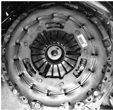
Abb. 2: Druckplatte ansetzen.
