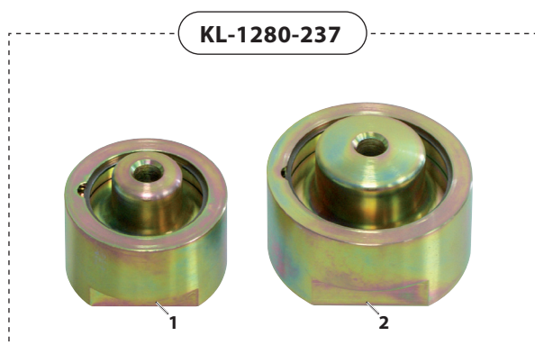
Abdeckungsstopfen mit Einschlagwerkzeug ansetzen.
