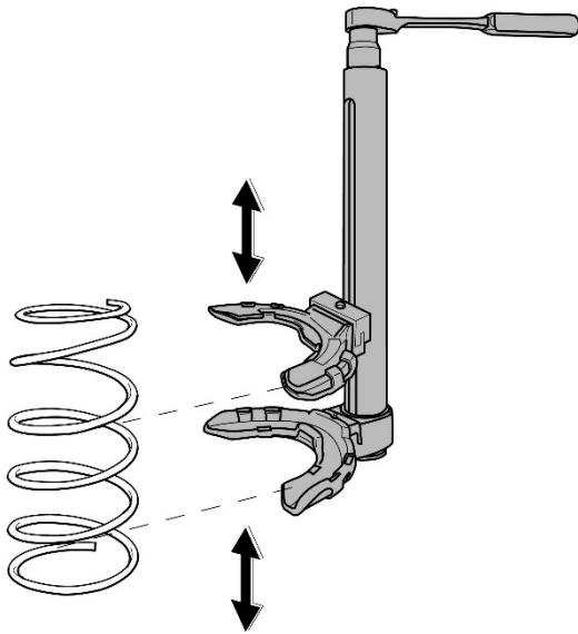
Abb. 23. Federspanngerät in die Feder einsetzen
