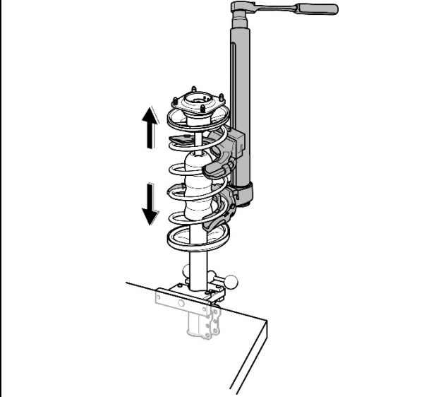
Abb. 30. Federspanngerät aus der Feder herausnehmen.
