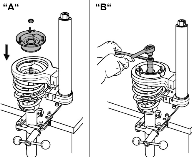
Abb. 38. Feder entspannen
