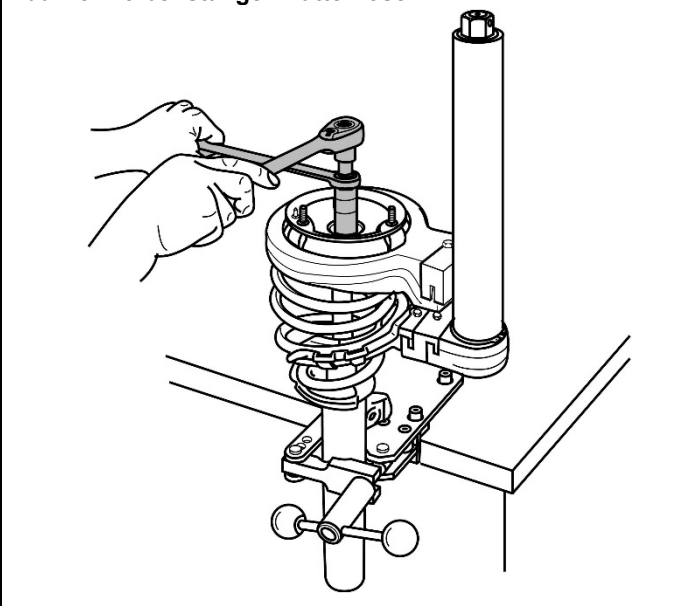
Abb. 18. Kolbenstangenmutter lösen
