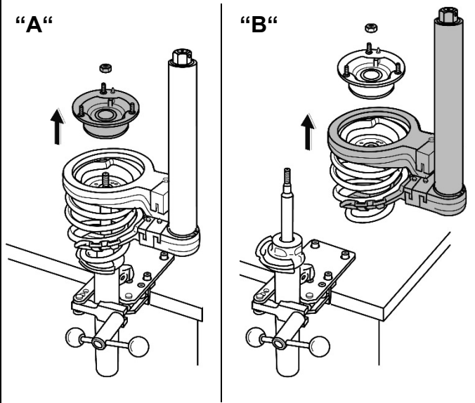
Abb. 20. Federhalter-Position markieren
