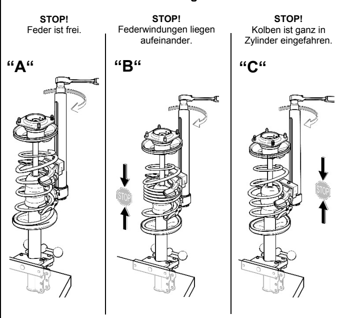
Abb. 12. Die Feder soweit spannen bis keine Spannung mehr auf der Kolbenstangenmutter ist.
