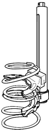
Abb. 27. Feder auf das Feder- oder Dämpferbein aufsetzen
