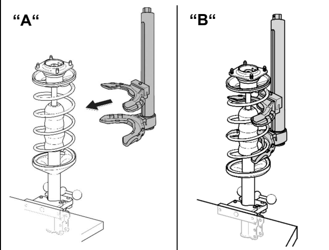
Abb. 11. Feder spannen
