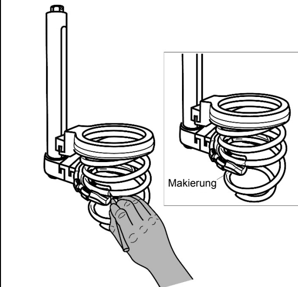
Abb. 21. Feder entspannen
