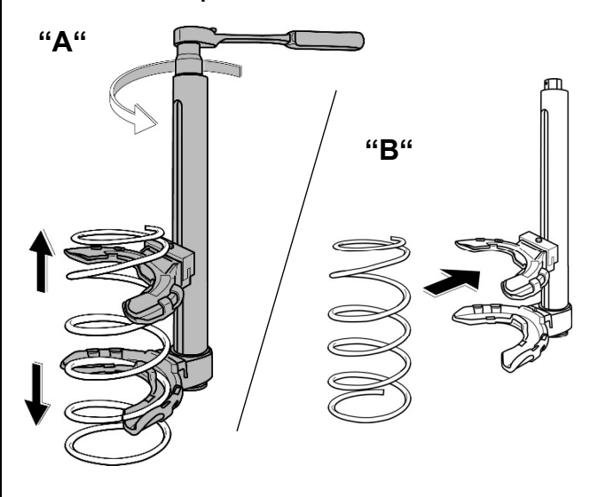
Abb. 15. Feder entspannen
