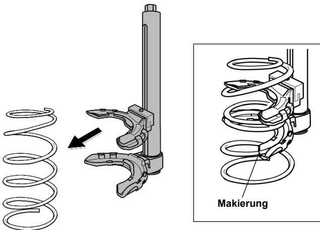
Abb. 24. Federspanngerät ist an der Feder angesetzt
