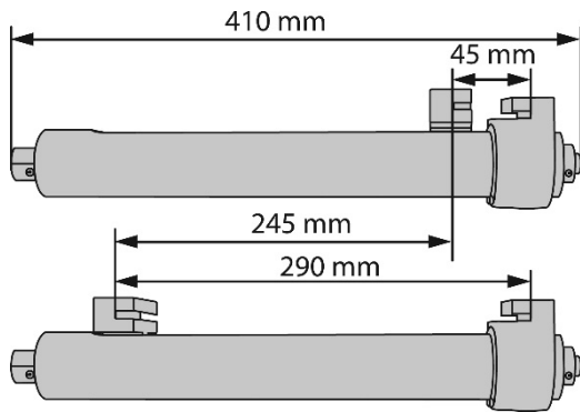
Abb. 1. Abmessungen KL-2000-100 (Spannzylinder)
