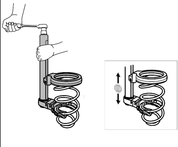
Abb. 21. Feder entspannen
