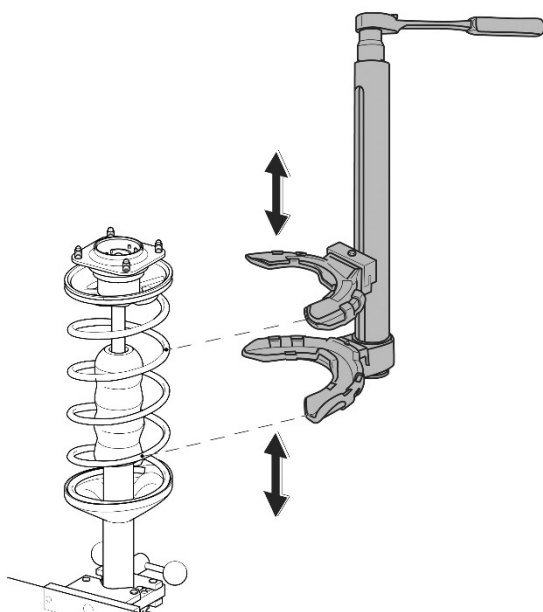
Abb. 9. Federspanngerät voreinstellen
