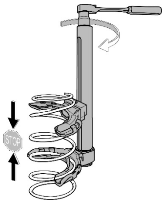
Abb. 26. Feder ist gespannt
