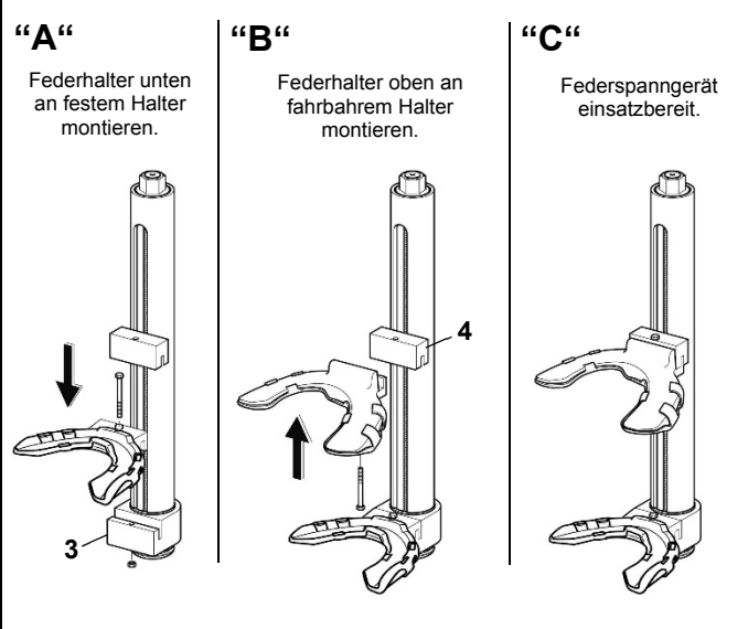
Abb. 6. Federhalter an Spannzylinder montieren (bei konischen Federn)
