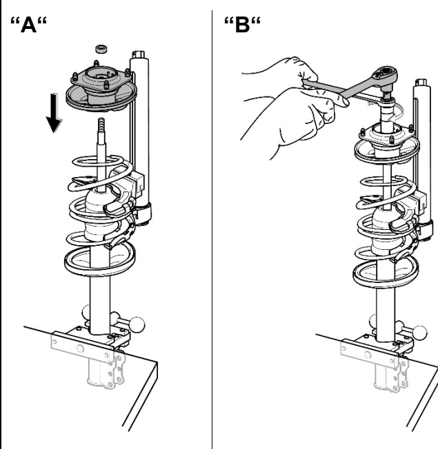
Abb. 29. Feder entspannen
