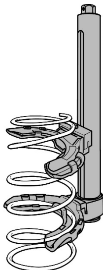
Abb. 24. Federspanngerät ist an der Feder angesetzt
