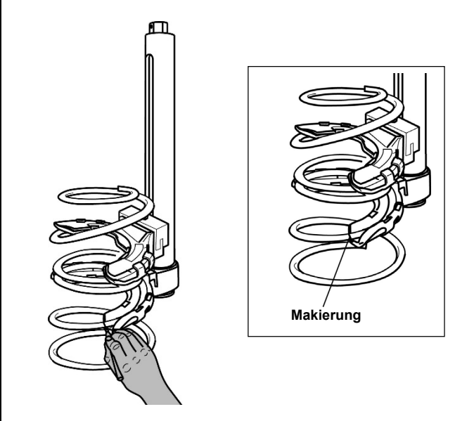
Abb. 15. Feder entspannen
