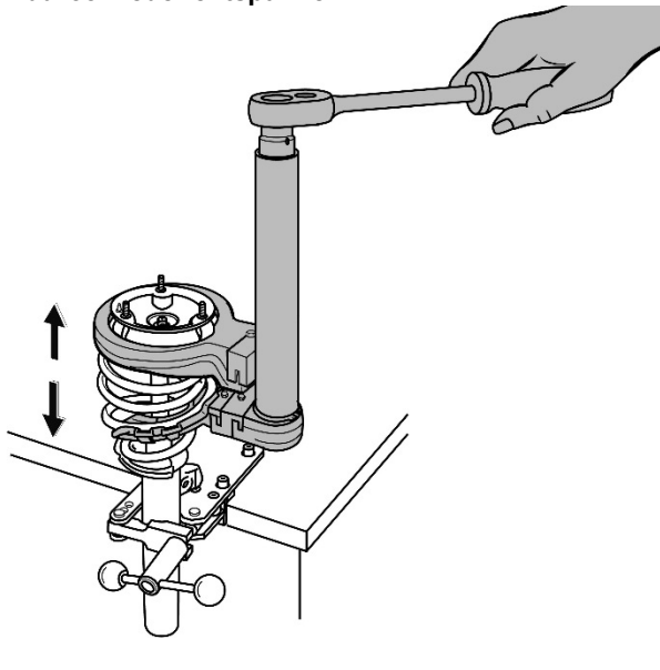
Abb. 38. Feder entspannen
