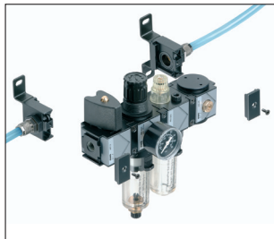
Schroefdraadverbindingsplaten met zelfklevende dichtringen (ook verkrijgbaar met bevestigingshoekstukken) voor een montagevriendelijke installatie in buisleidings- resp. slangensystemen.
