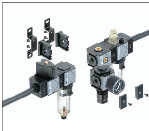
Bloqueo „comfort“. La solución rápida para el cambio de componentes y de la combinación con el módulo de unión (juntas de estanqueidad autoadhesivas) que reduce el tiempo de montaje.
