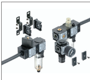
Comfortvergrendeling. De snelle vervanging van componenten of combinaties met verbindingmodule (dichtringen zijn zelfklevend) verkort de montagetijden.
