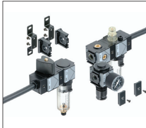
Komfortverblockung. Schneller Komponenten- oder Kombinationswechsel mit Verbindungsmodul (Dichtringe sind selbsthaftend) verkürzt Montagezeiten.
