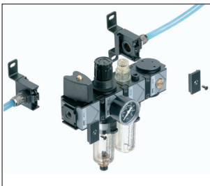
Gewindeanschlussplatten mit selbsthaftenden Dichtringen (auch mit Haltewinkel) für montagefreundliche Installation in Rohrleitungs- bzw. Schlauchsystemen.
