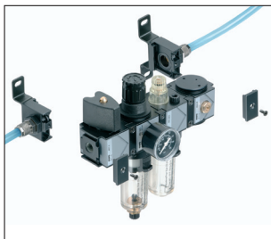
Plaques de connexion filetée avec joints auto-adhésifs (également disponible avec support de montage) pour l'installation à l'installation dans la tuyauterie et les systèmes de tuyau.
